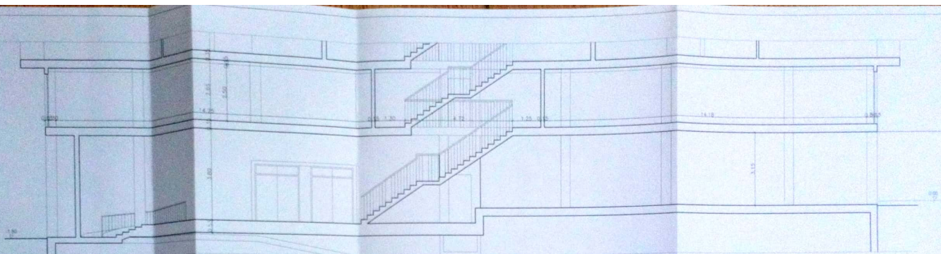
SECCION - ESTADO ACTUAL
